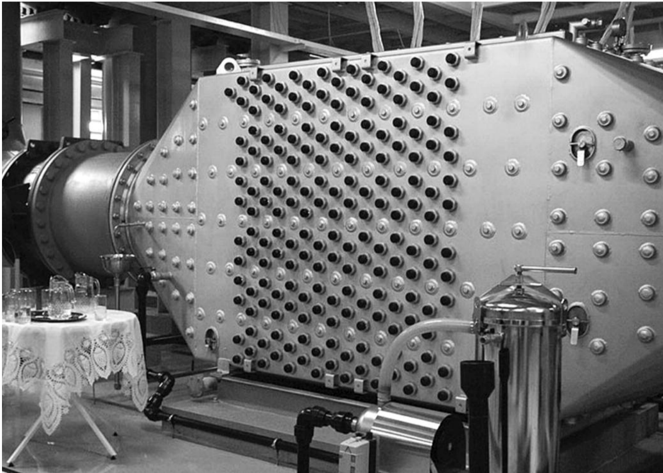
● НА ФОТО: УСТАНОВКА ПО УЛЬТРАФИОЛЕТОВОМУ ОБЕЗЗАРАЖИВАНИЮ ВОДЫ ОБОШЛАСЬ ГОРОДУ В 215 МЛН. РУБЛЕЙ
