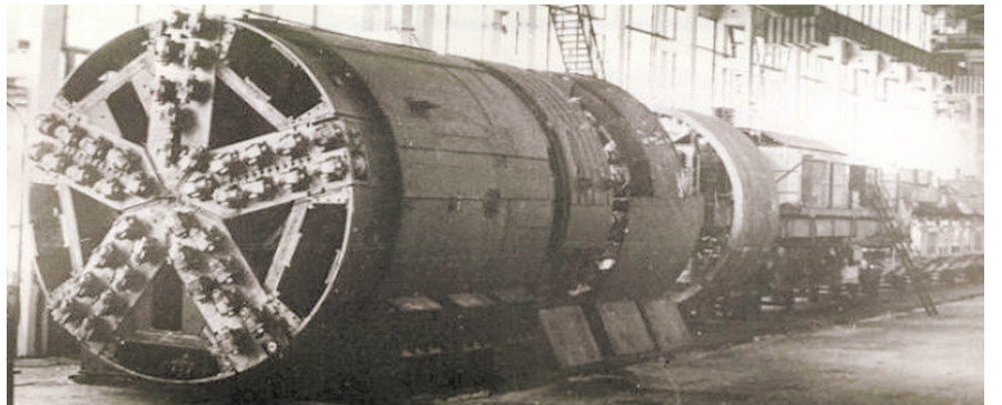
НА ФОТО: ЯСИНОВАТОВСКИЙ ТОННЕЛЕПРОХОДЧЕСКИЙ ЩИТ
