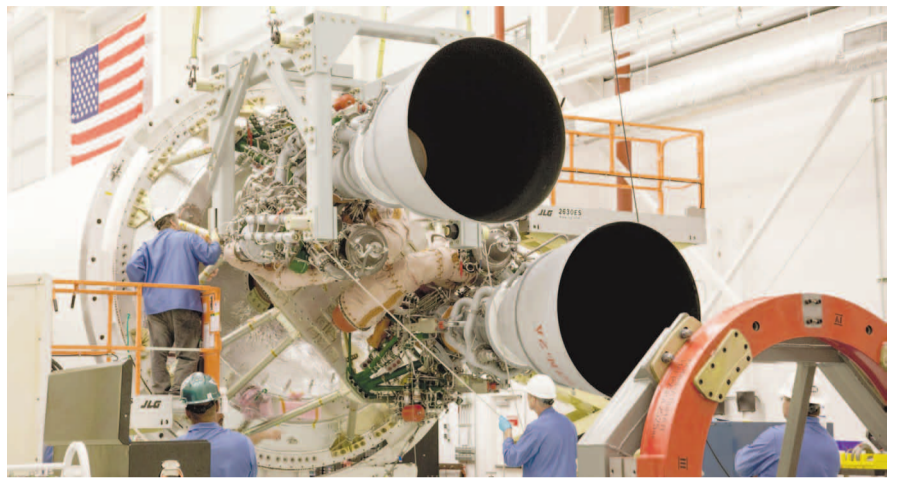
НА ФОТО: МОНТАЖ РОССИЙСКОГО ДВИГАТЕЛЯ РД-181 НА АМЕРИКАНСКУЮ РАКЕТУ-НОСИТЕЛЬ
